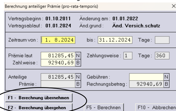
Abb.6: PRT – Berechnungsmaske
