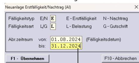
Abb.5: Auswahl Erstfälligkeit
